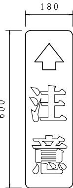
12 注意板 (S=1/10)
