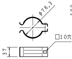
13 注意板取付バンド (S=1/6)
