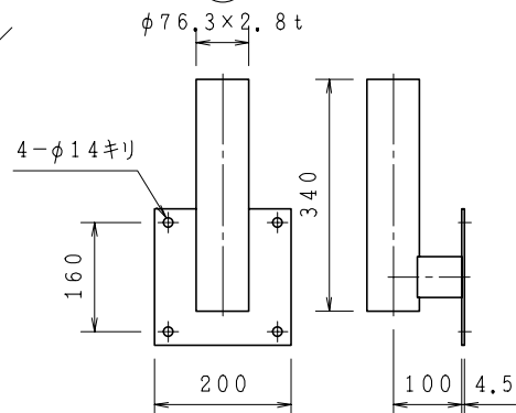
⑪ 壁面取付金具 (S=1/10)
