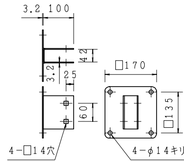
④ 裏板取付金具 (S=1/10)
