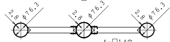
④ 裏板取付金具 (S=1/10)
