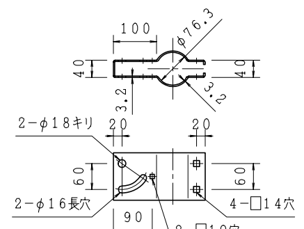
⑤ 支柱取付金具 (S=1/10)
