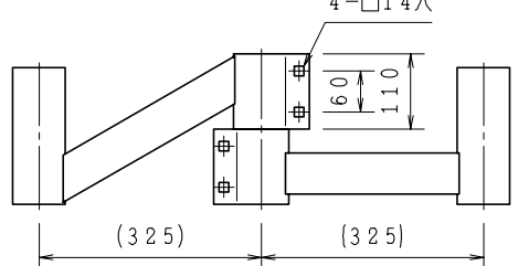
⑨ ⑩ 二面鏡用取付腕木 (S=1/10)
