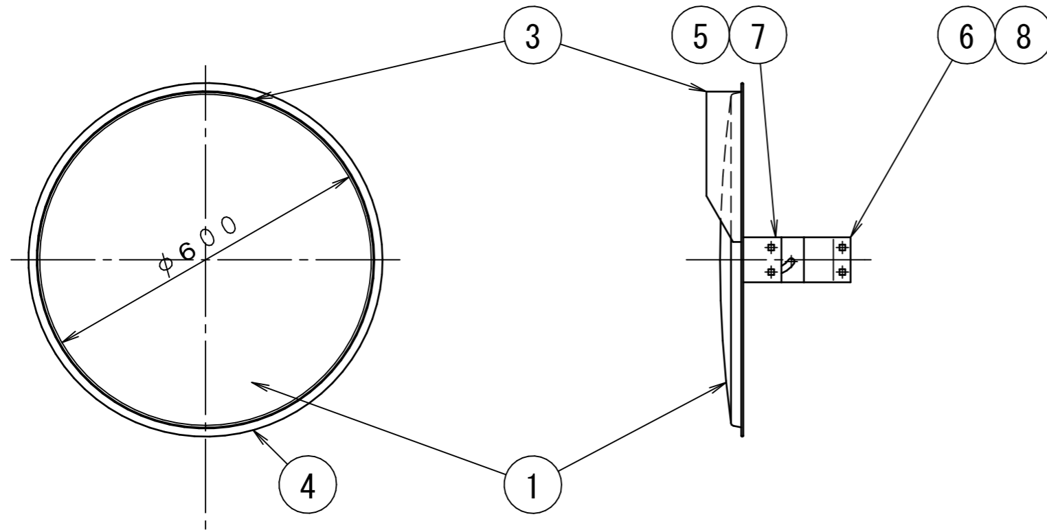
正面図
